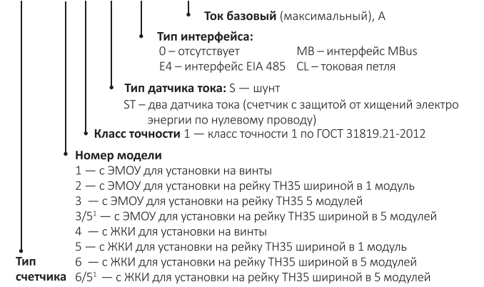
Рисунок 1. Структура условного обозначения счетчиков НЕВА 10
